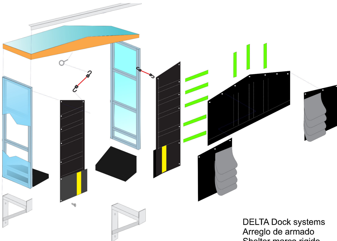
DELTA Dock systems Arreglo de armado Shelter Flexible
